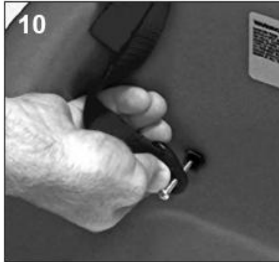
Montáž bezpečnostního pásu – kroky 9-11
